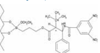
Structure du greffon \beta -GEM 1
